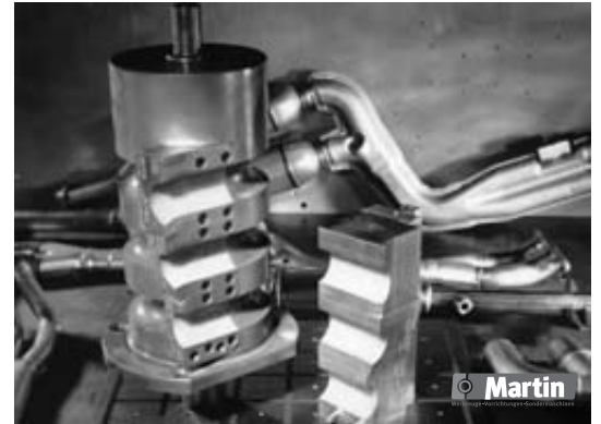
Rohr-Biegewerkzeuge
